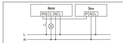
Master-Slave-Schaltung: Das Mastergerät schaltet angeschlossene Verbraucher je nach eingestellten Parametern. Die Slave-Geräte dienen nur der Bewegungserfassung und geben bei erkannter Bewegung einen Impuls an das Master-Gerät.
